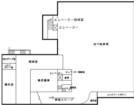
地階 (面積 1,536.09㎡)
