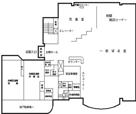
1階 (面積 1,601.04㎡)
